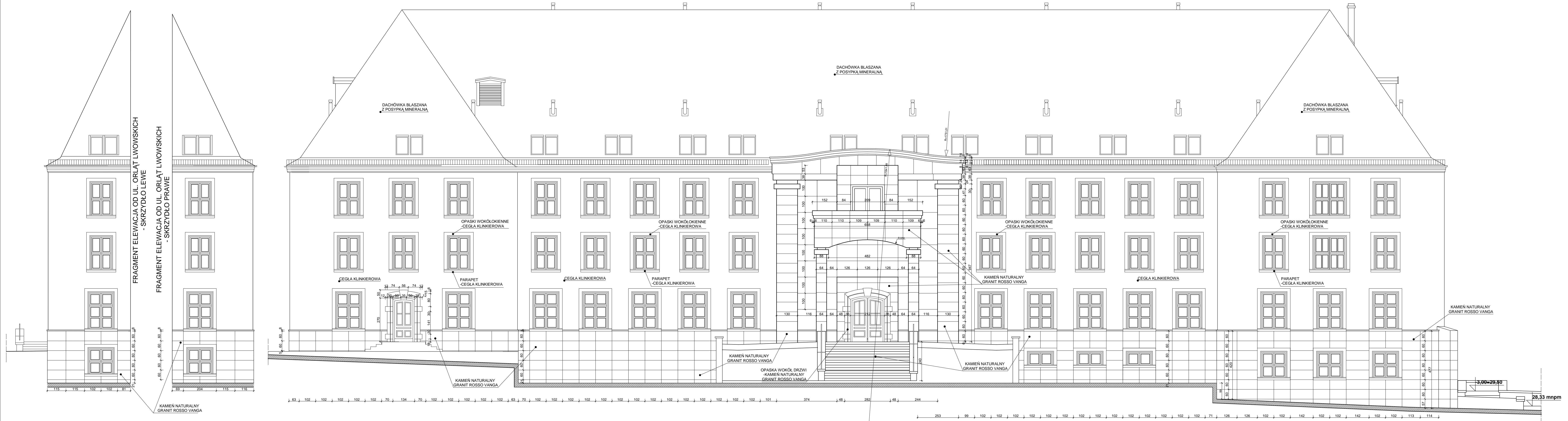
ELEWACJA OD UL. ORŁAT LWOWSKICH
