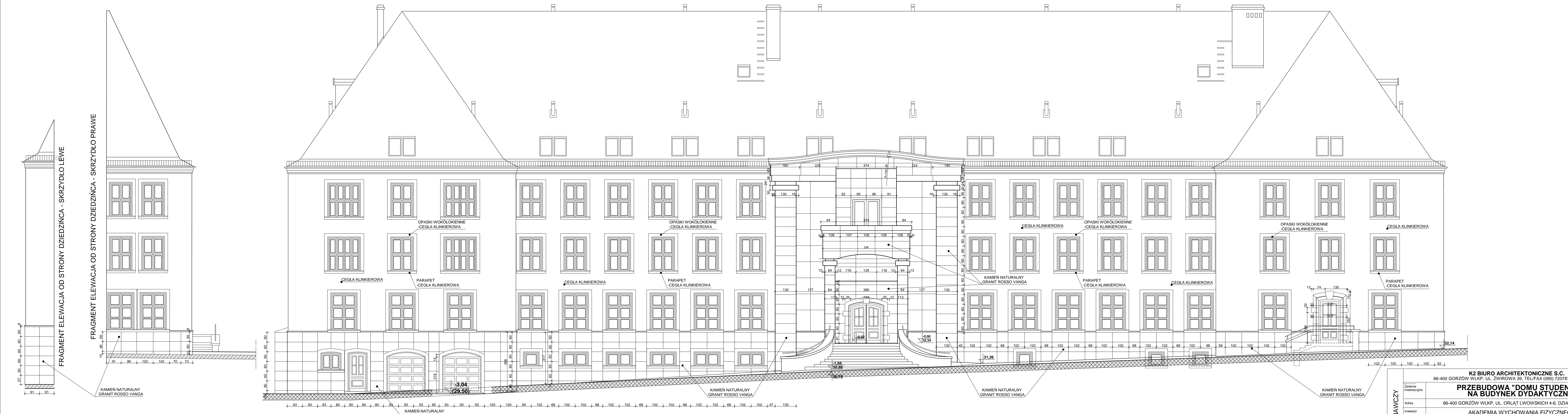
ELEWACJA OD STRONY DZIAŁKI
