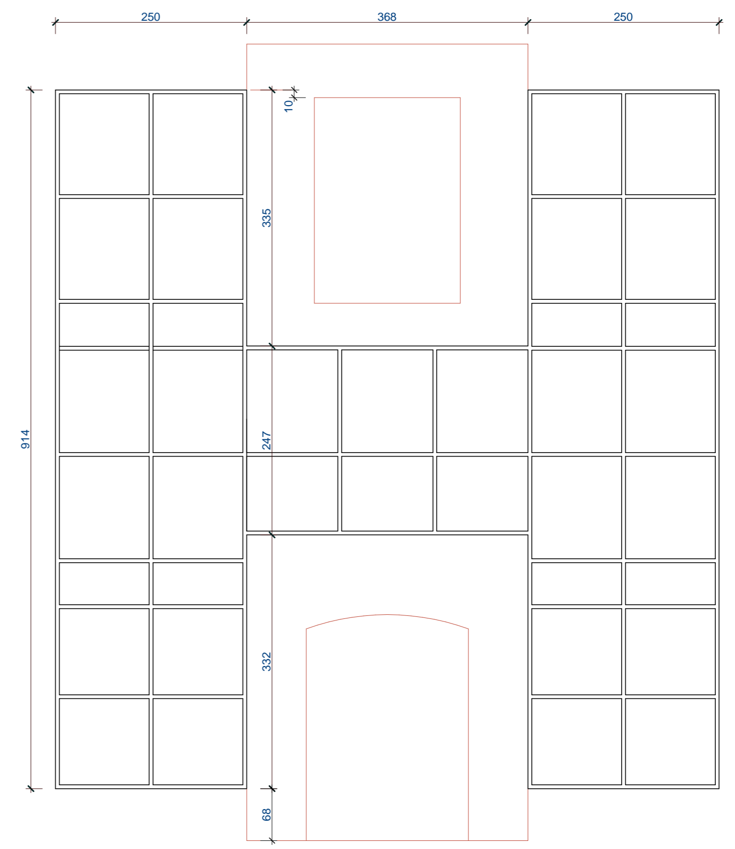
FASADA CAŁOSZKLANA OD UL. ORŁĄT LWOWSKICH
