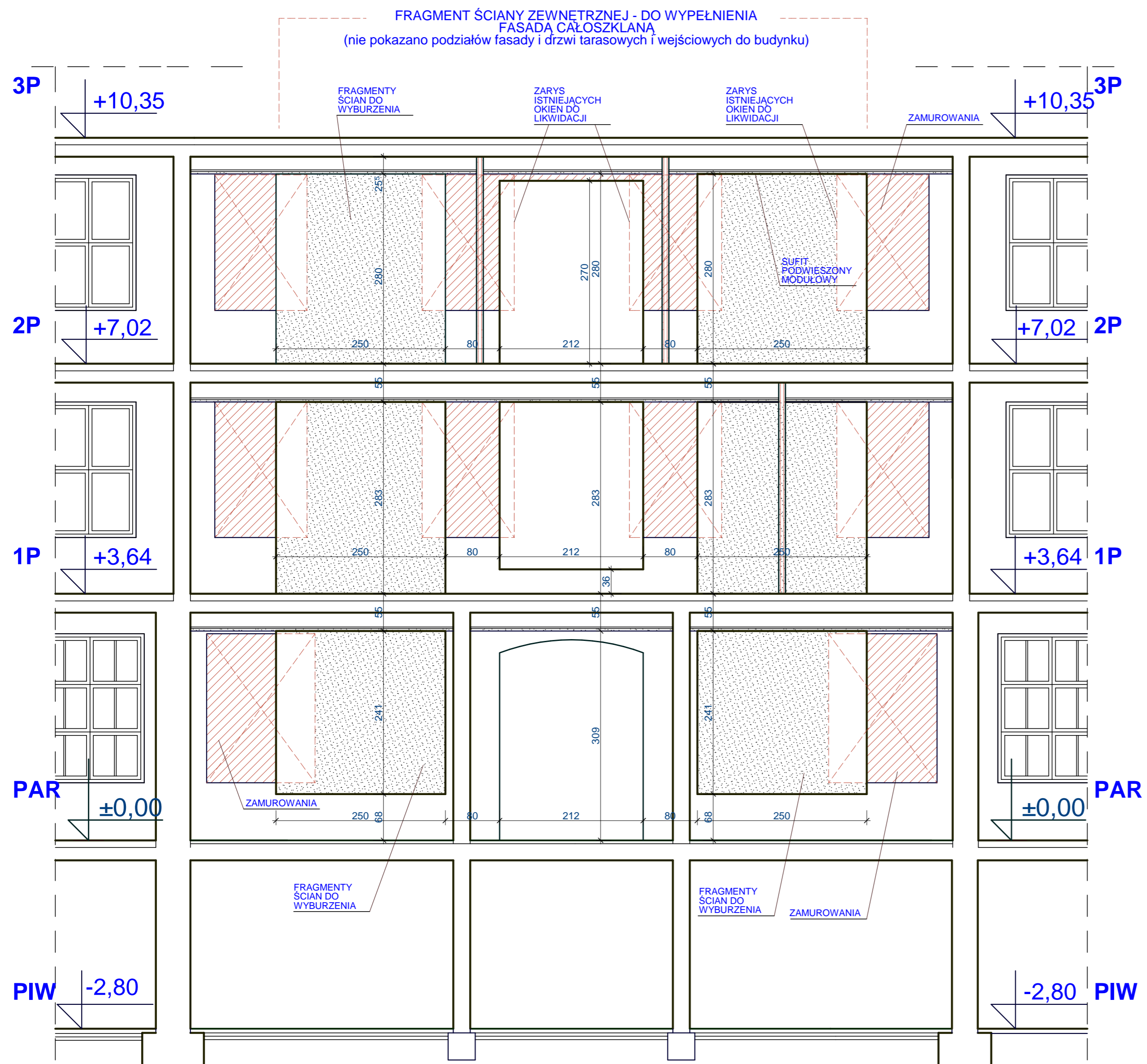
PRZEKRÓJ PODŁUŻNY Z WIDOKIEM Z WNĘTRZA BUDYNKU NA FASADĘ OD UL. ORŁĄT LWOWSKICH A4-A4
