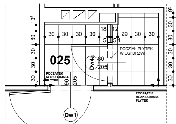
POMIESZCZENIE 025 WC
