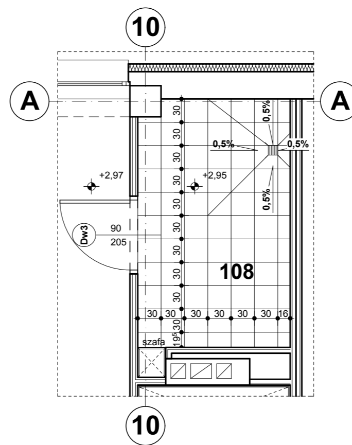
POMIESZCZENIE 108 ŁAZIENKA DLA NIEPEŁNOSPRAWNYCH
